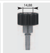
HV M22. Edelstahl. US-Version 14,88. Typ 05
