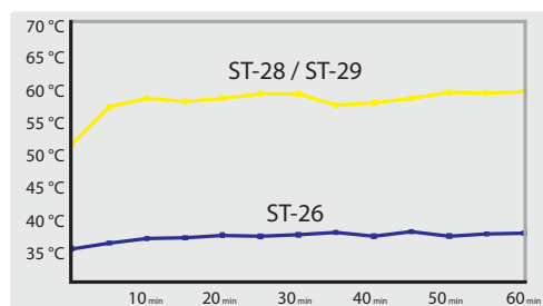
Oberflächentemperatur der Isolierungen ST-28, ST-29 und ST-26 bei einer Wassertemperatur von 90 °C.
