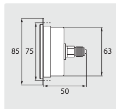
Ø 63 mm. 1/4" AG. Mit Frontplatte. Gehäuse Edelstahl. Eingang hinten
