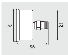
Ø 50 mm. 1/4" AG. Gehäuse Edelstahl. Eingang hinten
