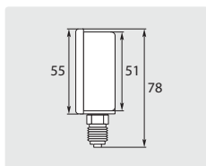
Ø 50 mm. 1/4" AG. Gehäuse Edelstahl. Eingang unten
