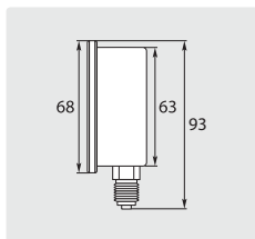
Ø 63 mm. 1/4" AG. Gehäuse Edelstahl. Eingang unten
