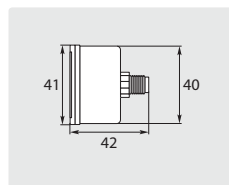
Ø 40 mm. 1/8" AG. Gehäuse Kunststoff. Eingang hinten
