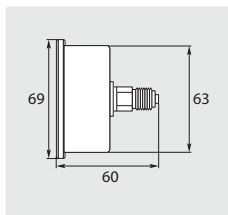
Ø 63 mm. 1/4" AG. Gehäuse Edelstahl. Eingang hinten
