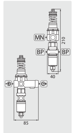
ST-261 Paneeleinbau mit Druckschalter
