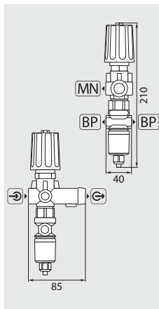
ST-261 mit Druckschalter 3-adrig
