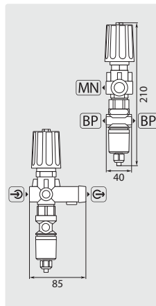
ST-261 mit Druckschalter 4-adrig
