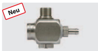
Tülle 9 mm : 1/2" AG dreh. : 1/2" IG. Edelstahl. Zum Einblasen von Druckluft. Max. 350 bar / 60 °C
