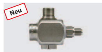
1/4" AG : 1/2" AG dreh. : 1/2" IG. Edelstahl. Zum Einblasen von Druckluft. Max. 350 bar / 60 °C
