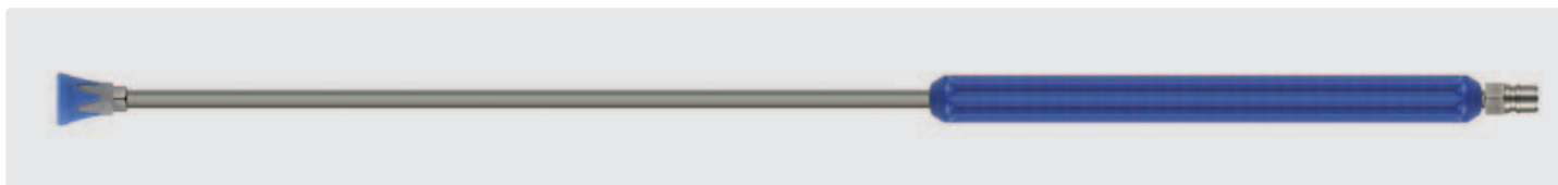
Stecknippel ST-45. Lanze aus Edelstahl mit umspritzter Isolierung und Düsenschutz ohne Düse. Max. 250 bar / 150 °C
